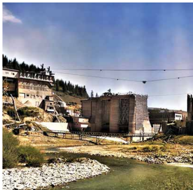
Stavbu vodného diela na Orave podnikli časté ničivé povodne, ale aj životne dôležitá potreba elektrifikácie štátu. Preto sa v tridsiatych rokoch minulého storočia začala výstavba dovtedy nevidanej diela podľa projektu architekta Pavla Andrika a stavba pokračovala v pôvodných zámeroch aj cez vojnu až po naplnenie priehrady a prifázovanie prvých blokov elektrárne pred sedemdesiatimi rokmi.
